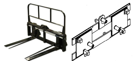
Kombigabel
