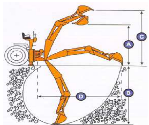
Heckbagger TS1-215
